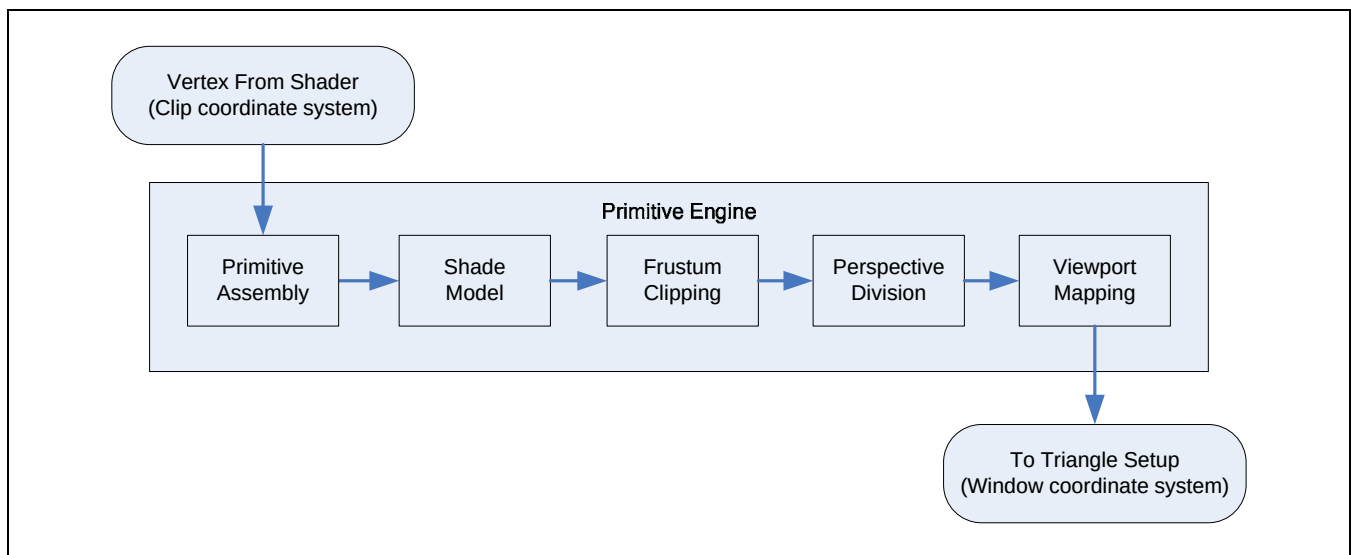
Figure 9.6- 12 PE Pipeline
